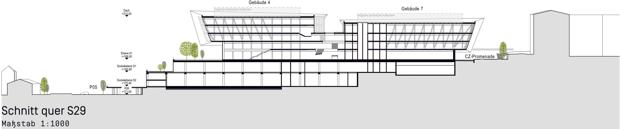
Ansicht Nord A-N Maßstab 1:1000
